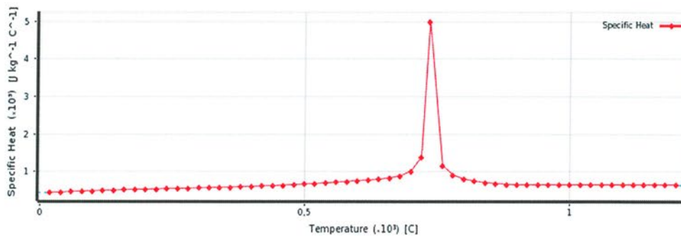
Diagramm 2: Stahl Spezifische Wärmekapazität
